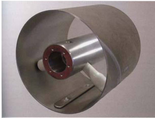
380 kV- gasisolierter Rohrleiter Kapseldurchmesser außen 517 mm, Leitungsdurchmesser außen 180 mm
